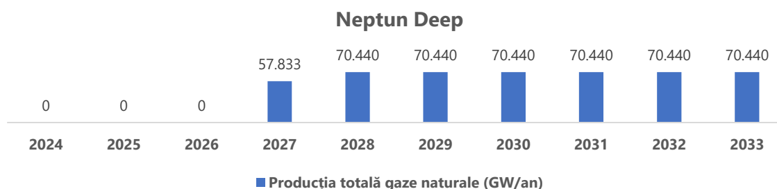
Grafic 14 – Prognoza producției de gaze naturale Neptun Deep în perioada 2024–2033
