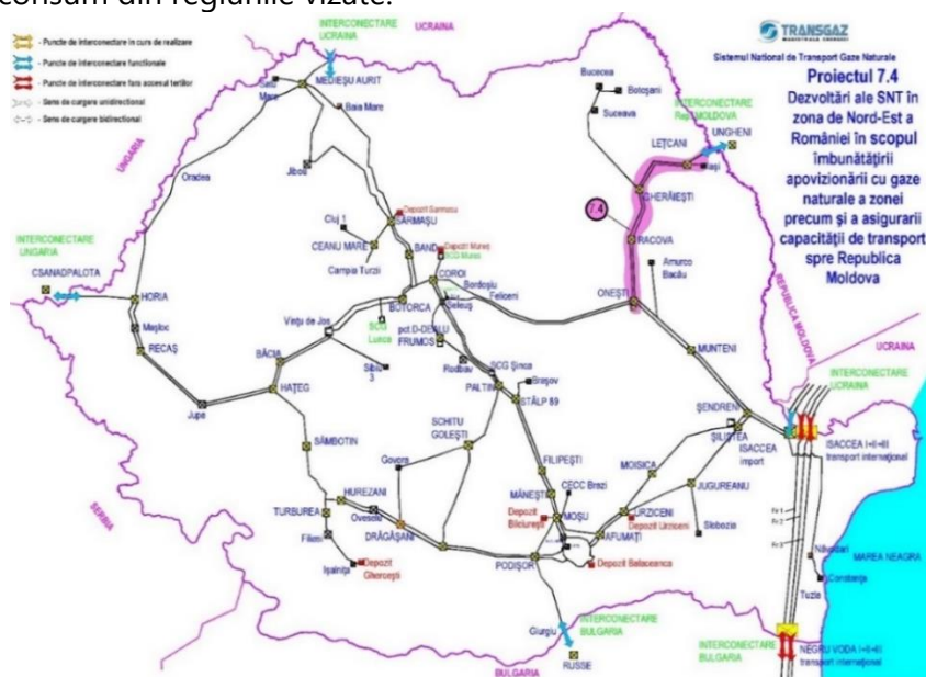
Figura 9-Dezvoltări ale SNT în zona de Nord-Est a României
