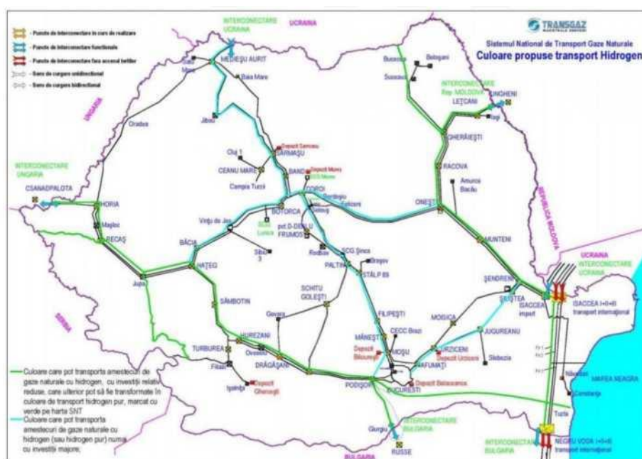
Figura 8 - Propunere a "coloanei vertebrale" a SNT pentru transportul hidrogenului, Sursă: Transgaz (2021)
