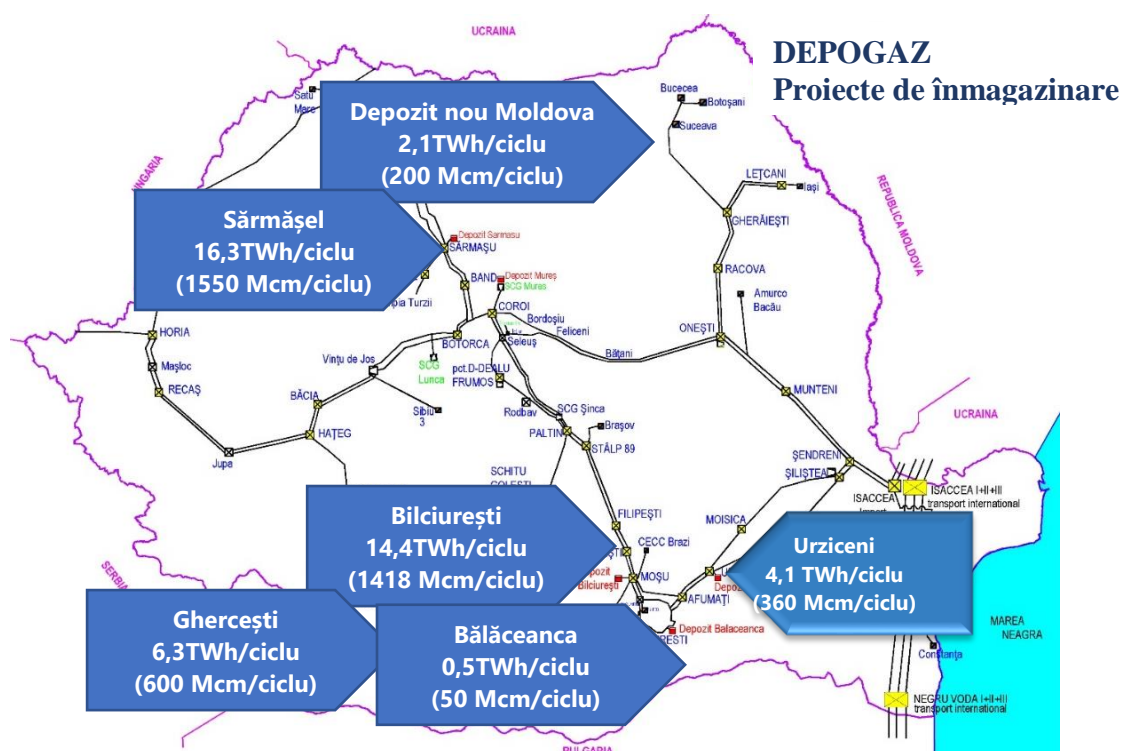
Figura 6 – Proiecte majore de înmagazinare gaze naturale – Depogaz
