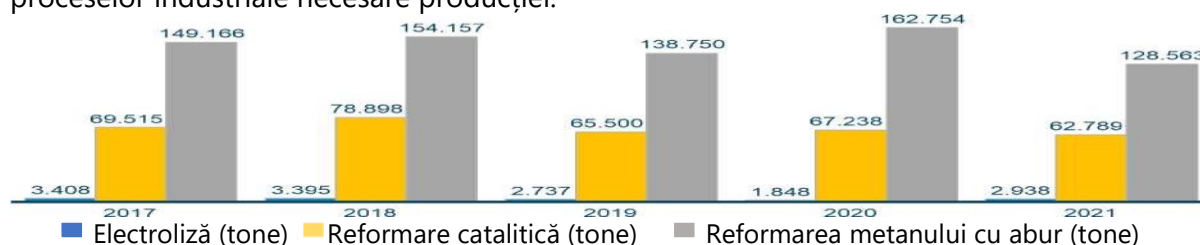
Grafic 17 - Producția de hidrogen pe tipuri de tehnologii, exprimată în tone, pentru perioada 2017-2021, Sursă: Analiză Horvath pe baza informațiilor primite de la principalii producători/consumatori de hidrogen din industrie (Februarie 2022)
