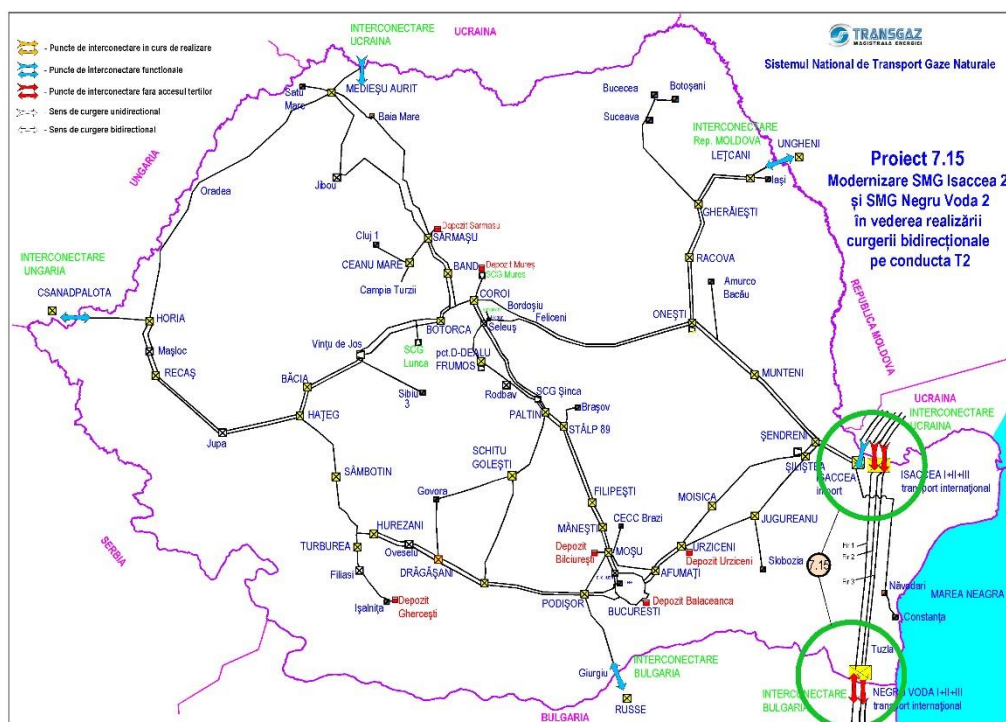
Figura 20 - Modernizare SMG Isaccea 2 și SMG Negru Vodă 2 în vederea realizării curgerii bidirecționale pe conducta T2
