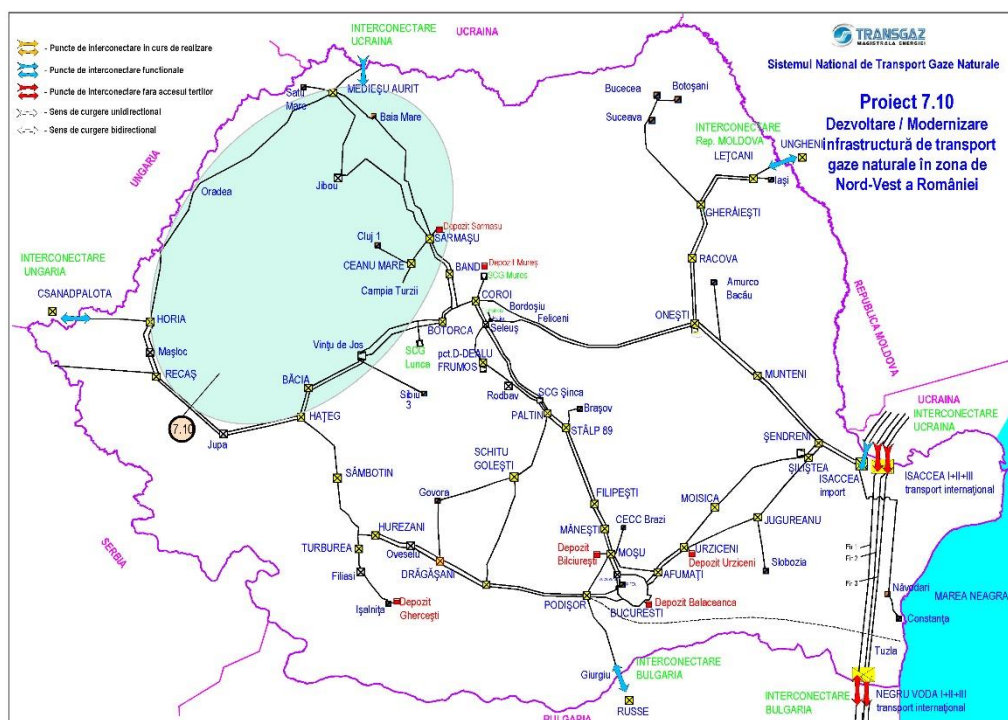
Figura 17- Dezvoltarea/Modernizarea infrastructurii de transport gaze naturale în zona de Nord-Vest a României
