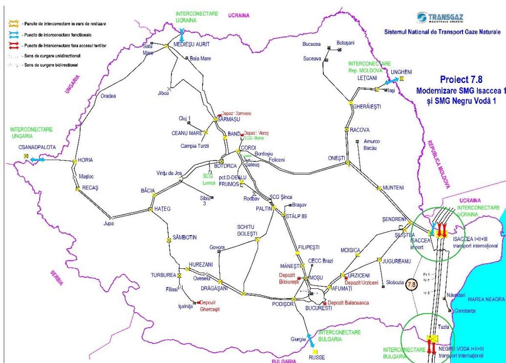
Figura 15 - Modernizare Negru Vodă 1
