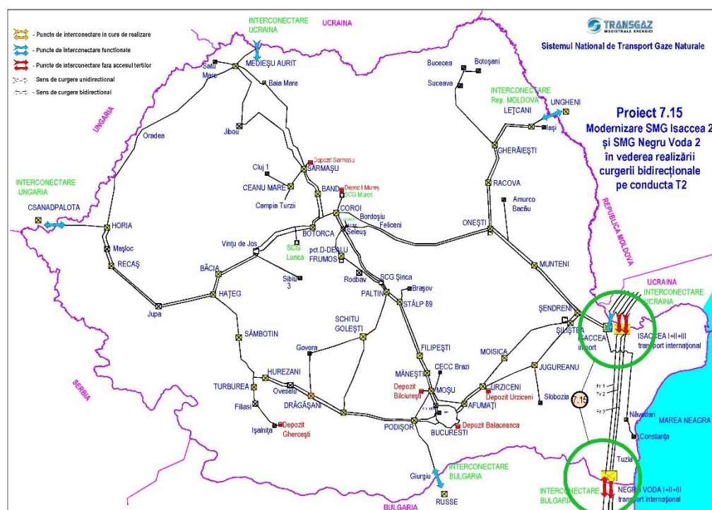
Figura 21- Modernizare SMG Isaccea 3 și Negru Voda 3 în vederea realizării curgerii bidirecționale pe conducta T3
