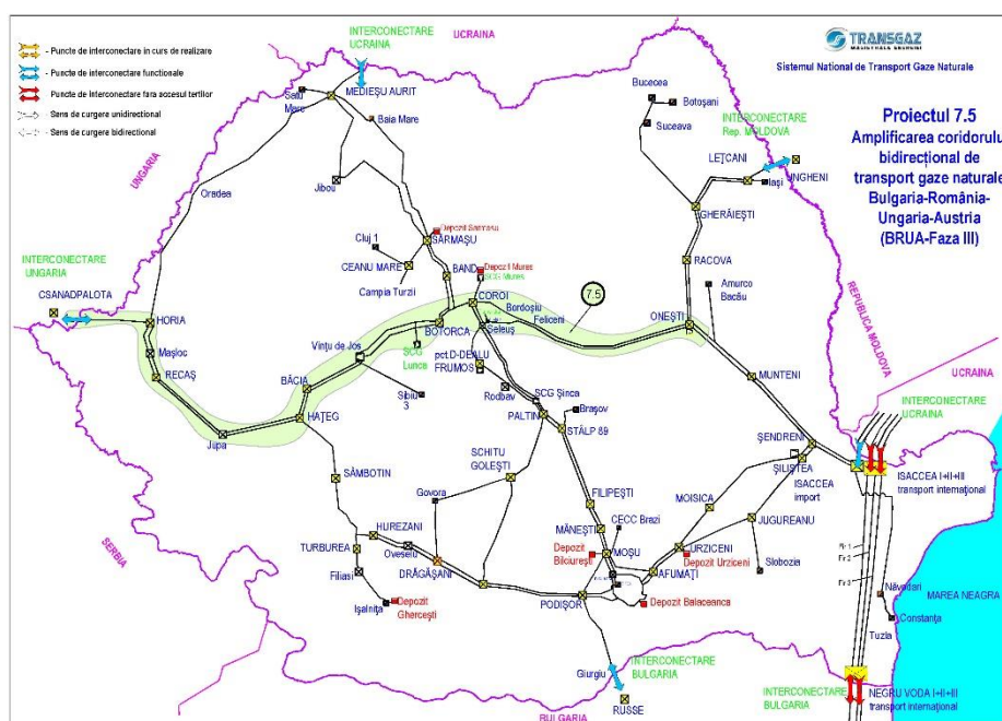
Figura 12- Dezvoltare BRUA -Faza III
