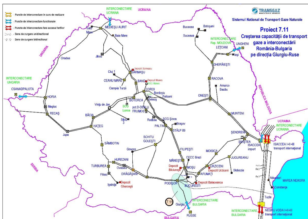
Figura 18- Creșterea capacității de transport gaze naturale a interconectării România-Bulgaria pe direcția Giurgiu-Ruse
