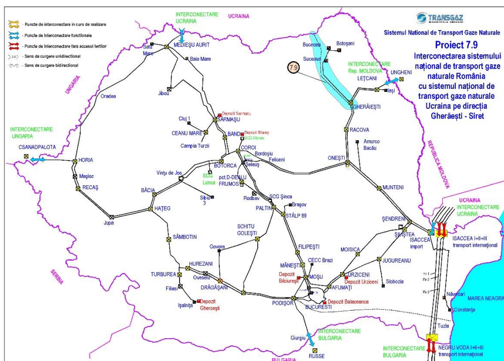
Figura 16 - Interconectarea sistemului național de transport gaze naturale România cu sistemul național de transport gaze naturale Ucraina pe direcția Gherăești-Siret
