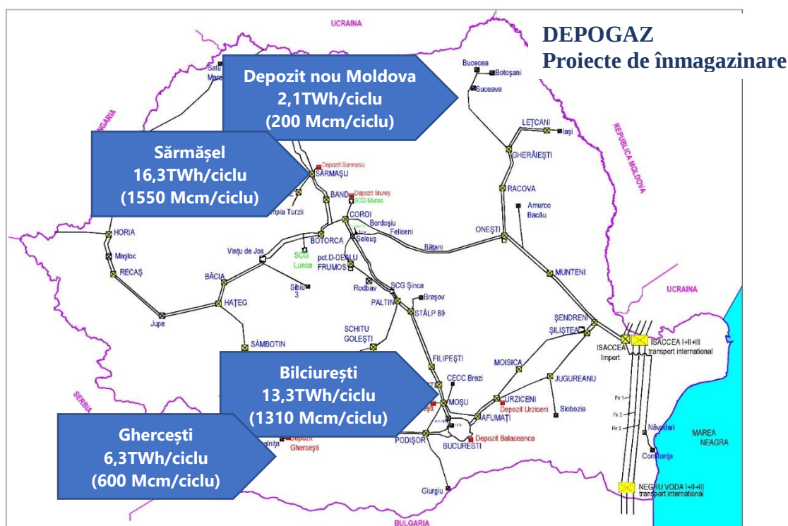
Figura 23 – Proiecte majore de înmagazinare gaze naturale – Depogaz
