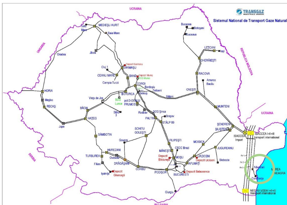
Figura 22 - Interconectarea SNT la Terminal GNL amplasat la malul Mării Negre
