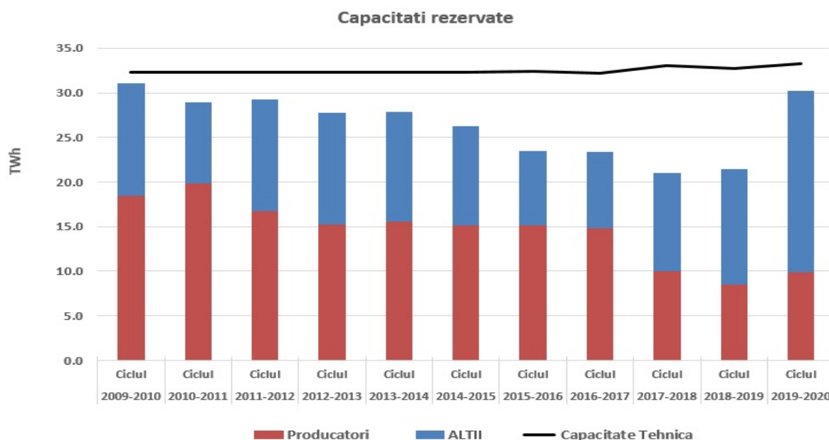
Grafic 19– Capacități rezervate în perioada 2009-2020
