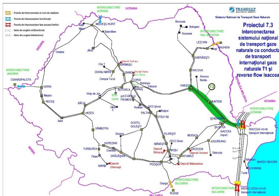
Figura 26 - Harta proiectului major de dezvoltare pentru interconectarea SNT cu conducta de transport internațional Tranzit 1 și reverse flow Isaccea
