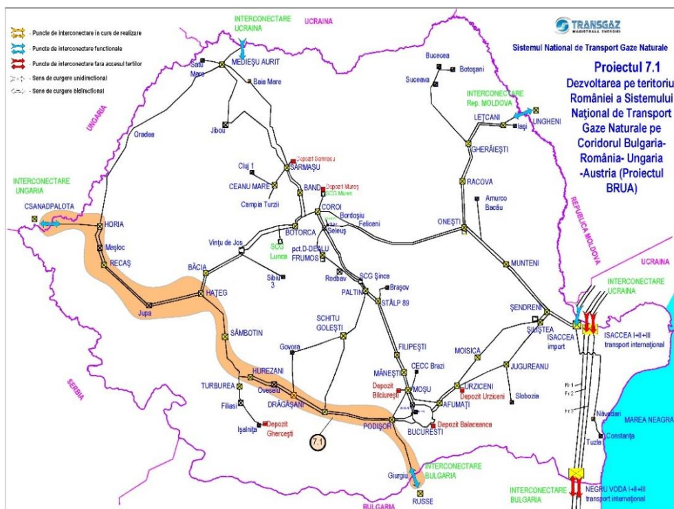
Figura 25 – Harta proiectului major de dezvoltare al coridorului Bulgaria-România-Ungaria-Austria – Faza I
