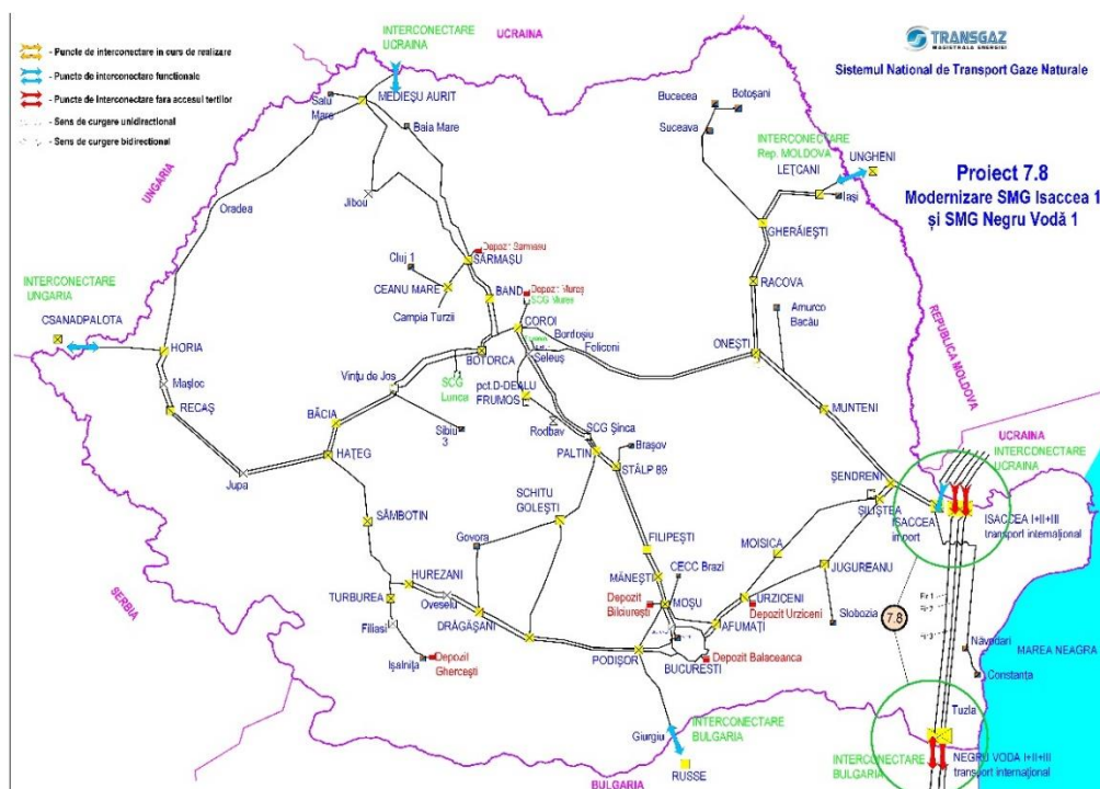
Figura 15 - Modernizare SMG Negru Vodă 1
