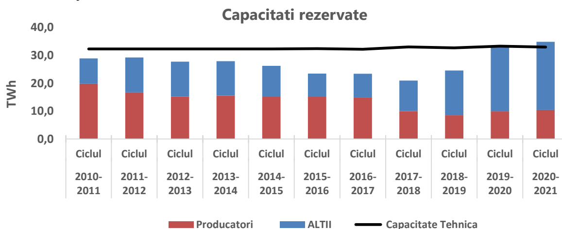
Grafic 19– Capacități rezervate în perioada 2010-2021
