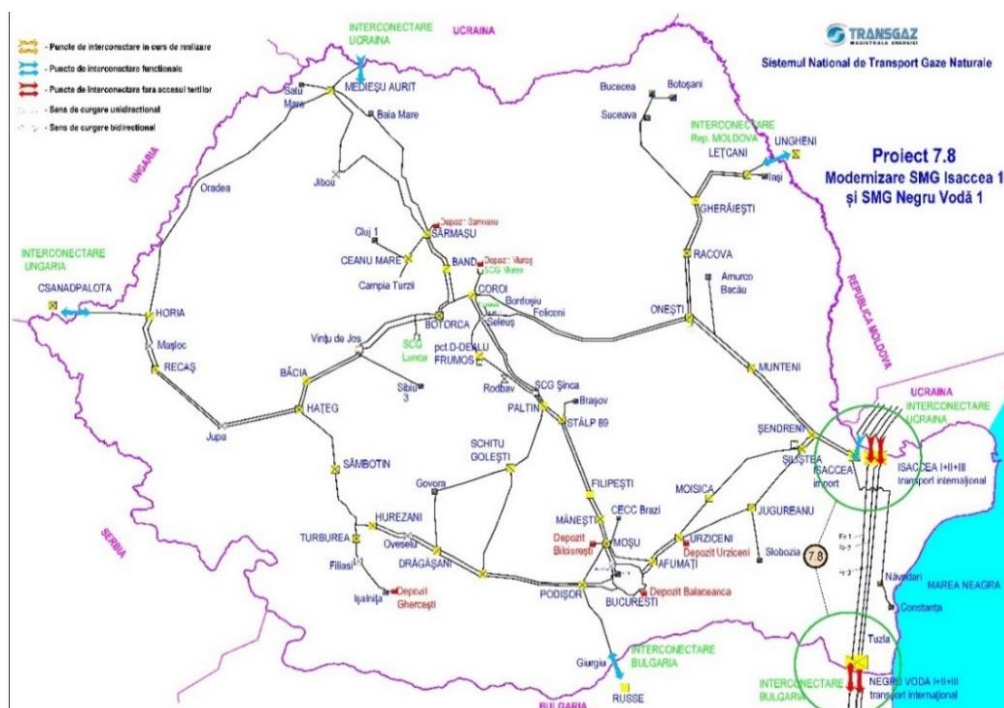
Figura 27 - Modernizare SMG Isaccea 1 și Negru Vodă 1
