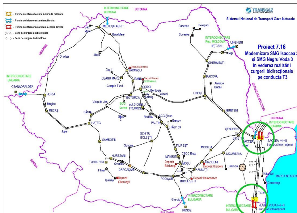
Figura 21- Modernizare SMG Isaccea 3 și SMG Negru Voda 3 în vederea realizării curgerii bidirecționale pe conducta T3
