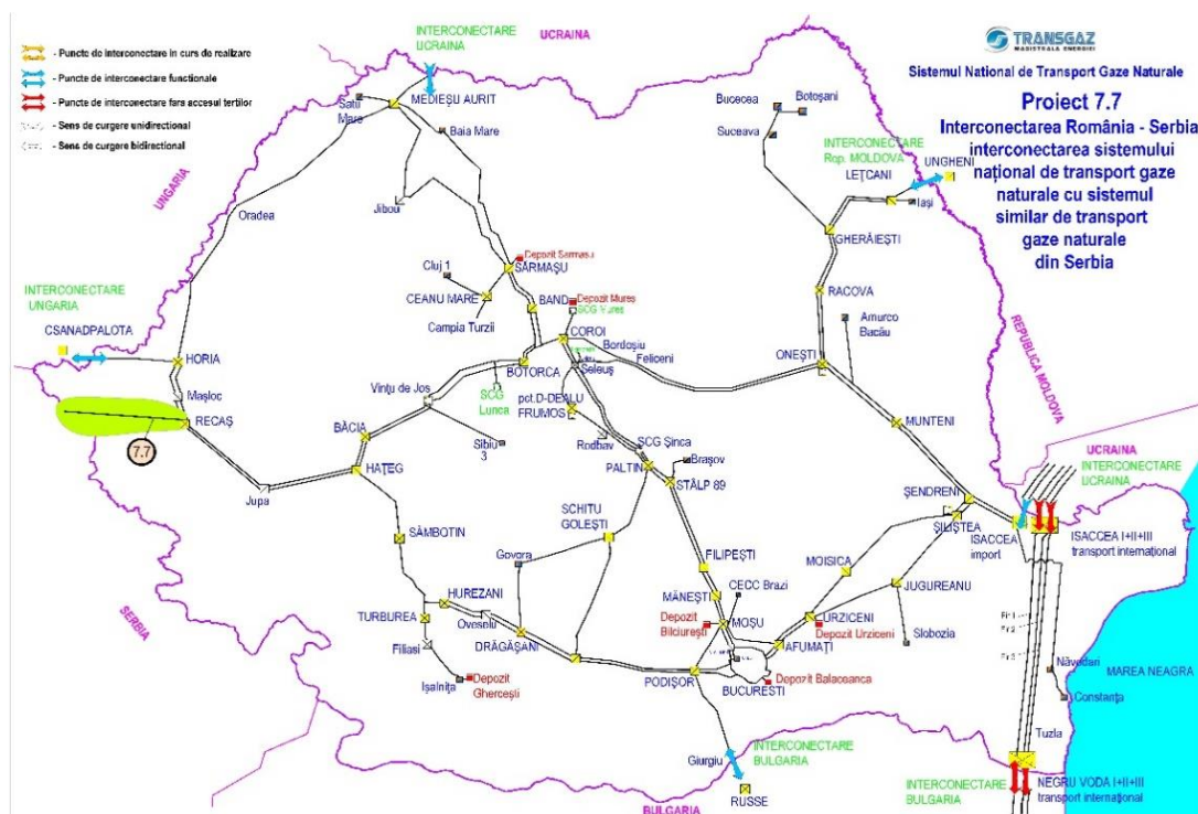
Figura 14 - Interconectarea SNT cu Serbia pe direcția Recaş-Mokrin
