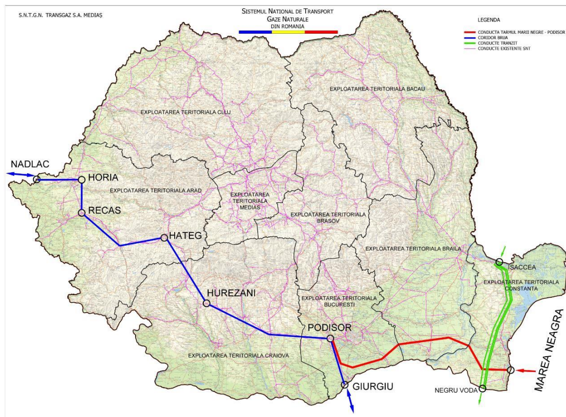
Reprezentare traseu conductă Țărmul Mării Negre - Podișor
