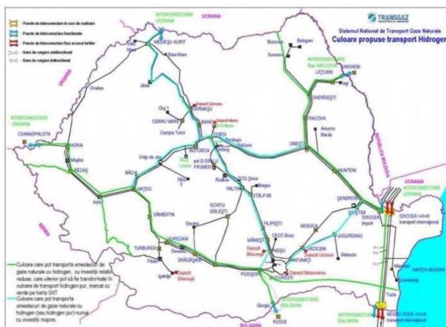
Figura 8 - Propunere a "coloanei vertebrale" a SNT pentru transportul hidrogenului, Sursă: Transgaz (2021)
