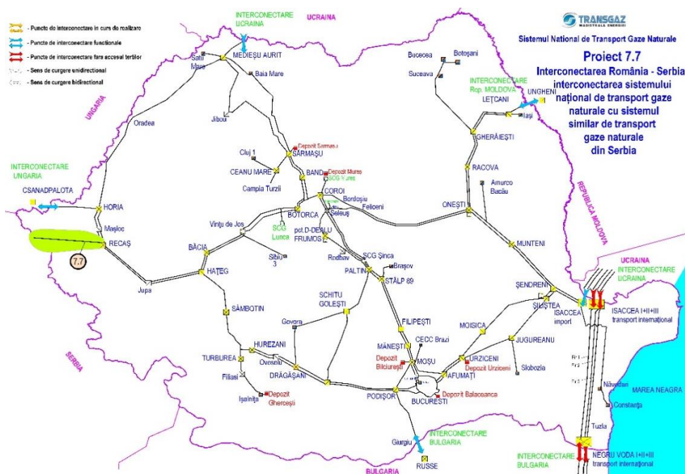
Figura 14 - Interconectarea SNT cu Serbia pe direcția Recaş–Mokrin
