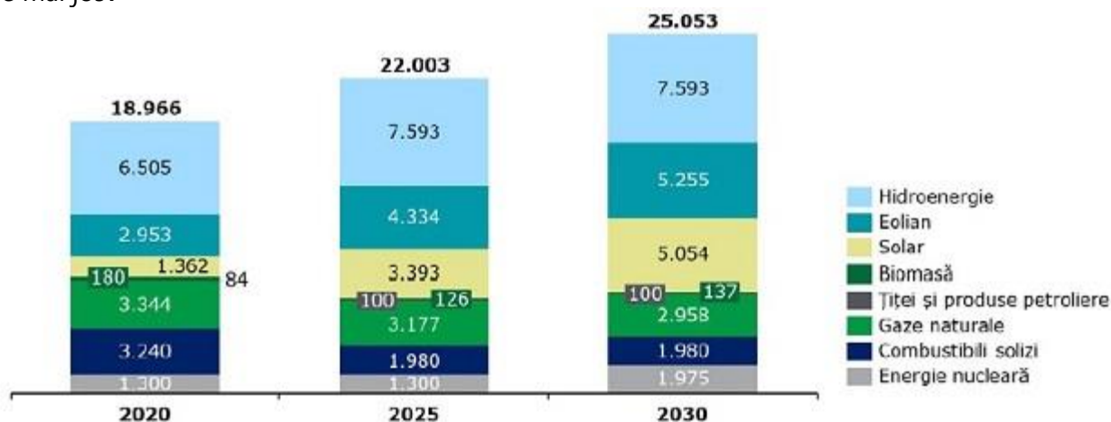
Traietoria orientativă a capacității nete instalate, pe surse în perioada 2020-2030, [MW]
