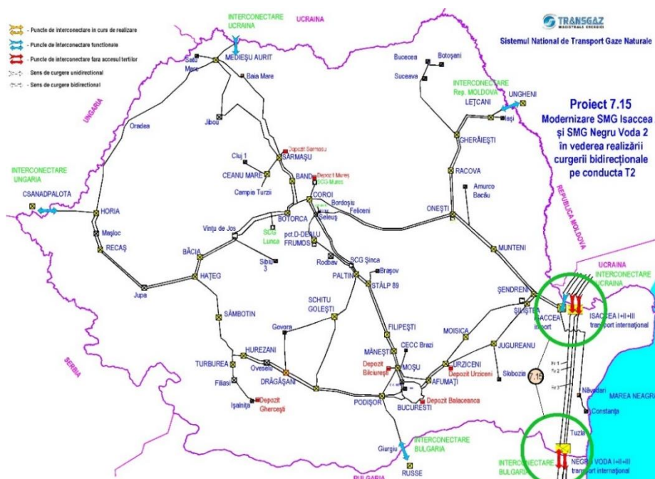
Figura 18 - Modernizare SMG Isaccea 2 și SMG Negru Voda 2 în vederea realizării curgerii bidirecționale pe conducta T2
