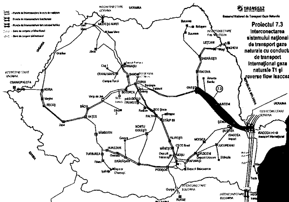
Figura 2 - Harta proiectului major de dezvoltare pentru interconectarea SNT cu conducta de transport internațional Tranzit 1 și reverse flow Isaccea
