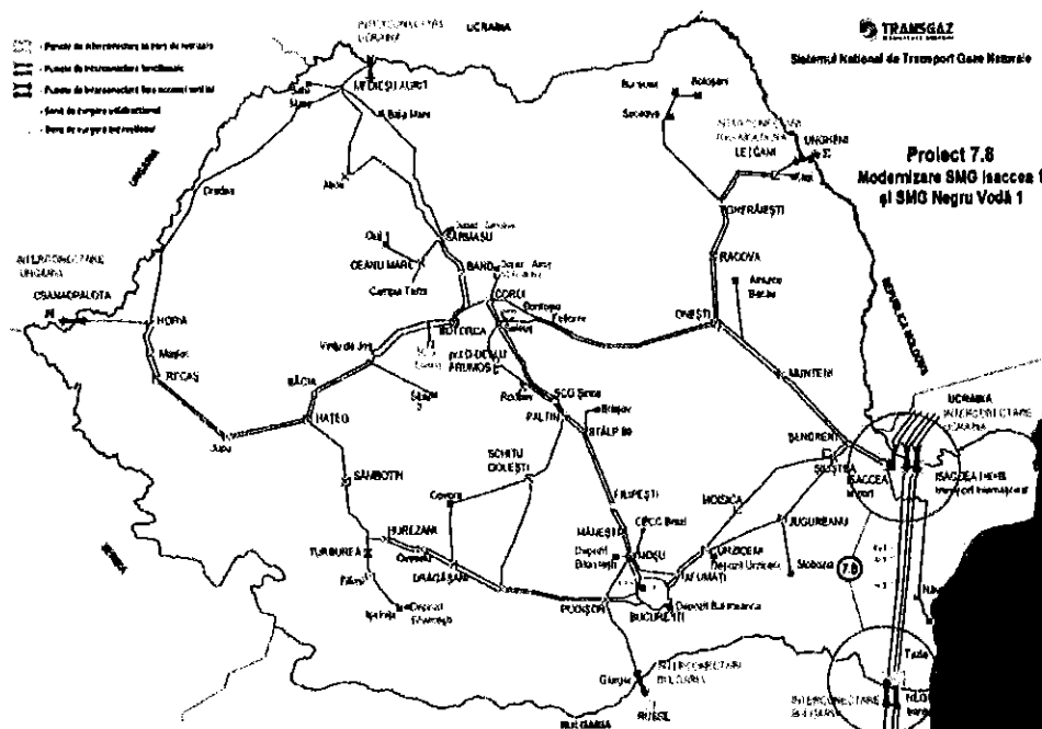
Figura 3- Modernizare SMG Isaccea 1 și Negru Vodă 1
